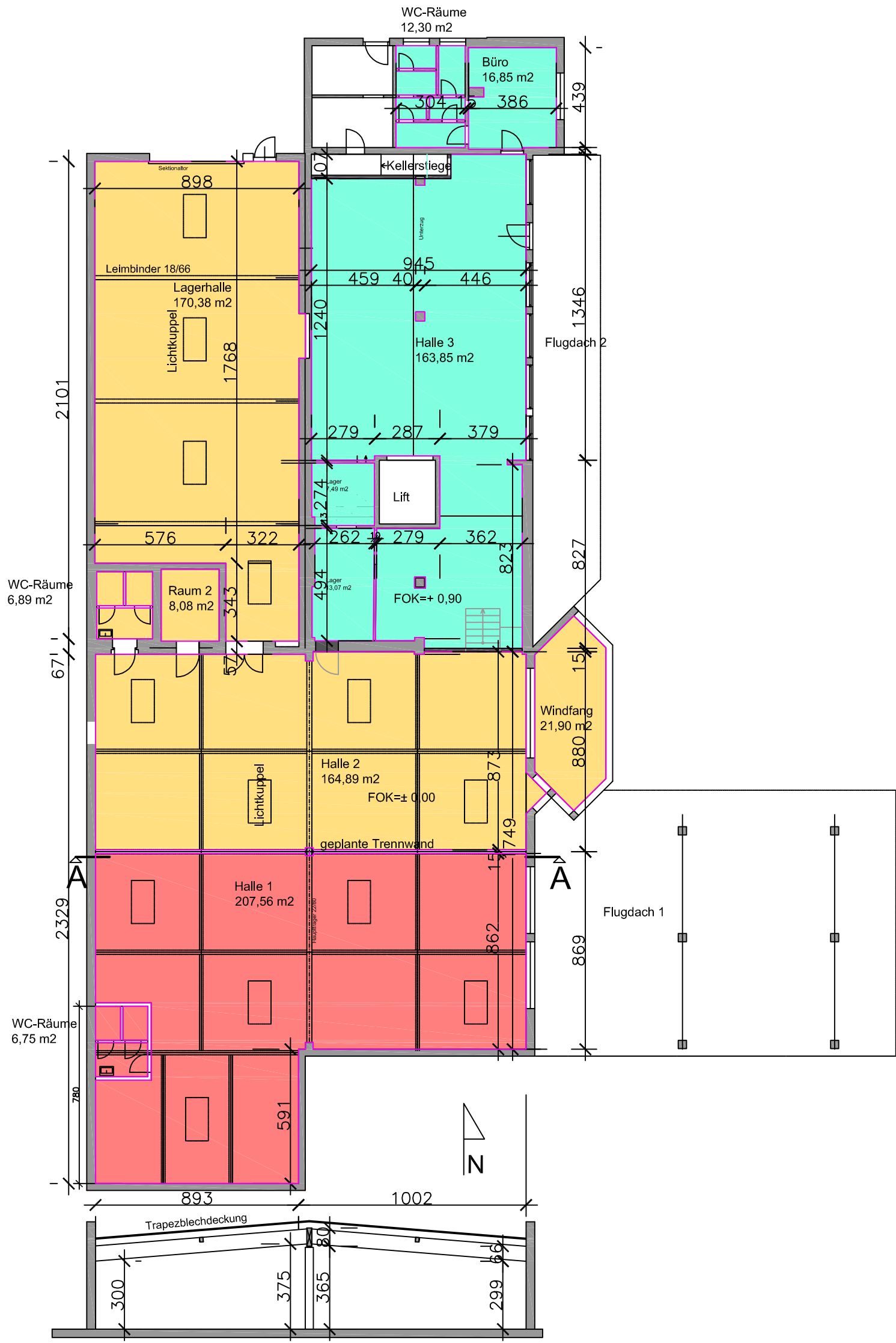
Schnitt A-A
